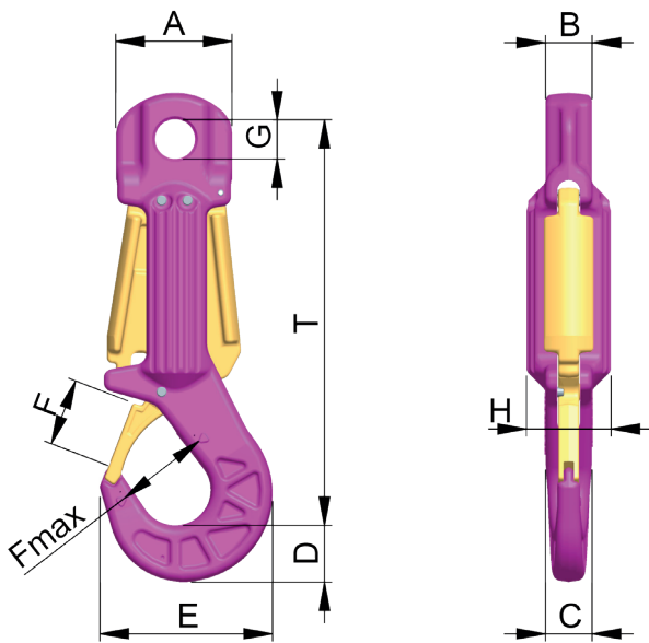
Fig. 15: Dimensions
